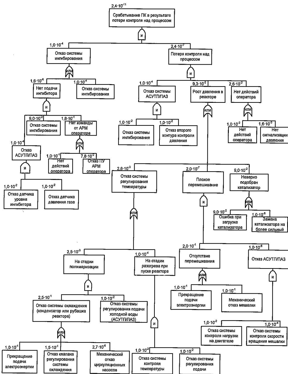
Рисунок 8-1. Пример дерева отказов для химических реакторов
